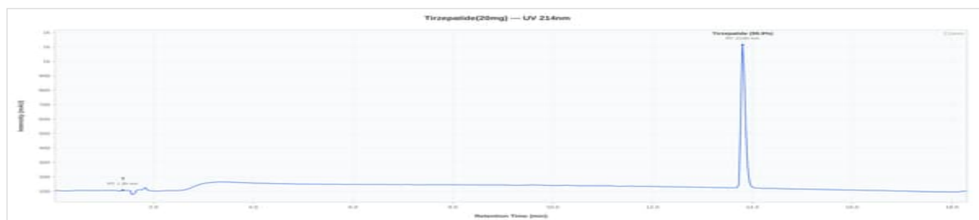
Tirzepatide 20mg - FS-2606-TZP20-001: UV Chromatogram
